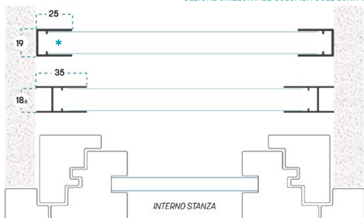
SEZIONE ORIZZONTALE COLOMBA SOLE LUNA V
