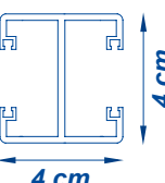
Guida accoppiata
